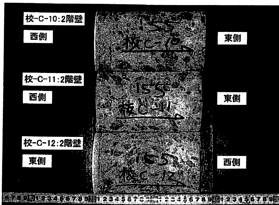
写真-4.a 搬入された供試体
