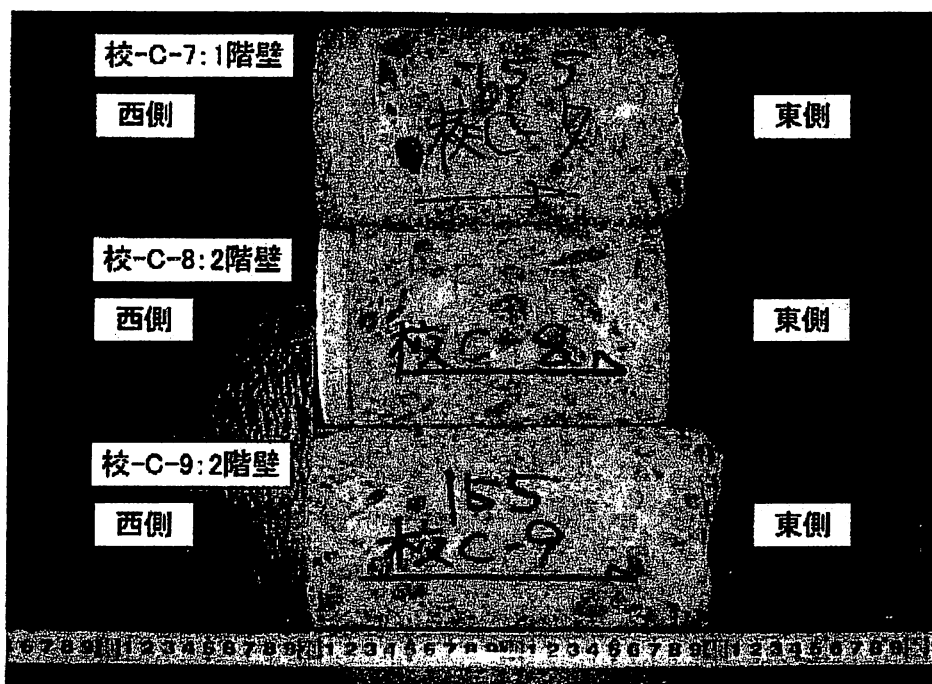
写真-3.a 搬入された供試体
