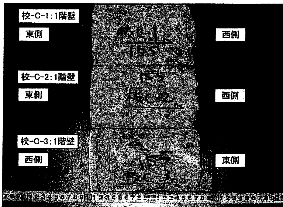
写真-1.a 搬入された供試体
