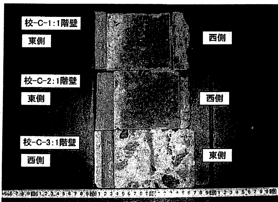
写真-1.b 中性化の状況
