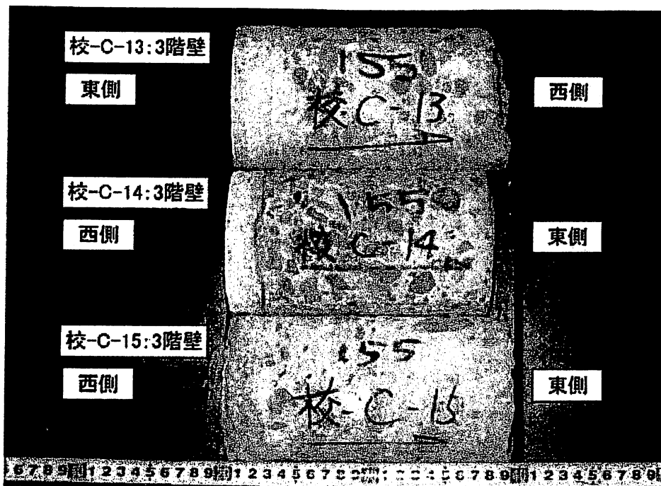
写真-5.a 搬入された供試体
