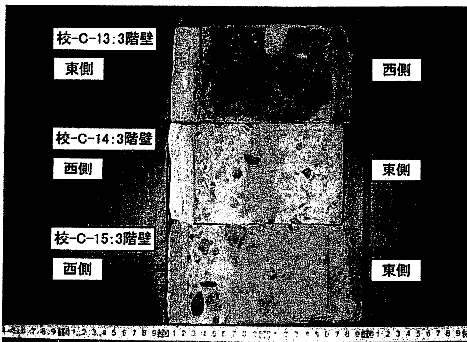
写真-5.b 中性化の状況
