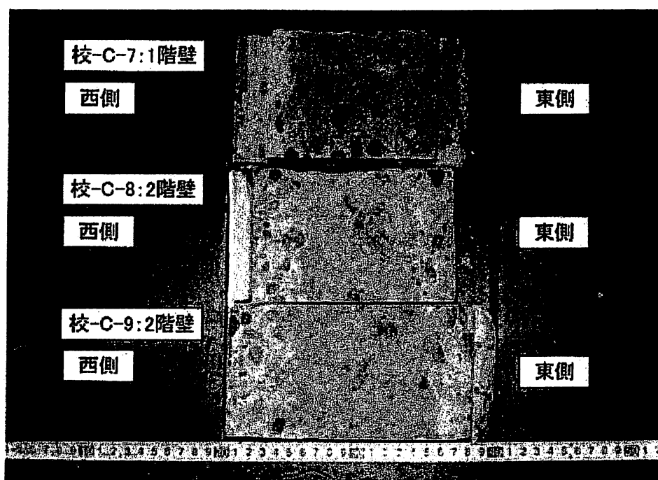
写真-3.b 中性化の状況
